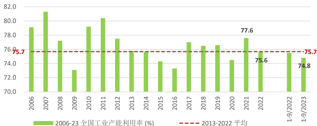
图表 6：全国工业产能利用率（%）－产能过剩导致产能利用率下降，对资本密集型行业不利，单位固定成本难以摊销下降
