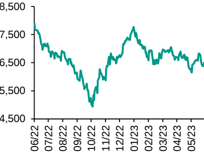
标普500走势图
